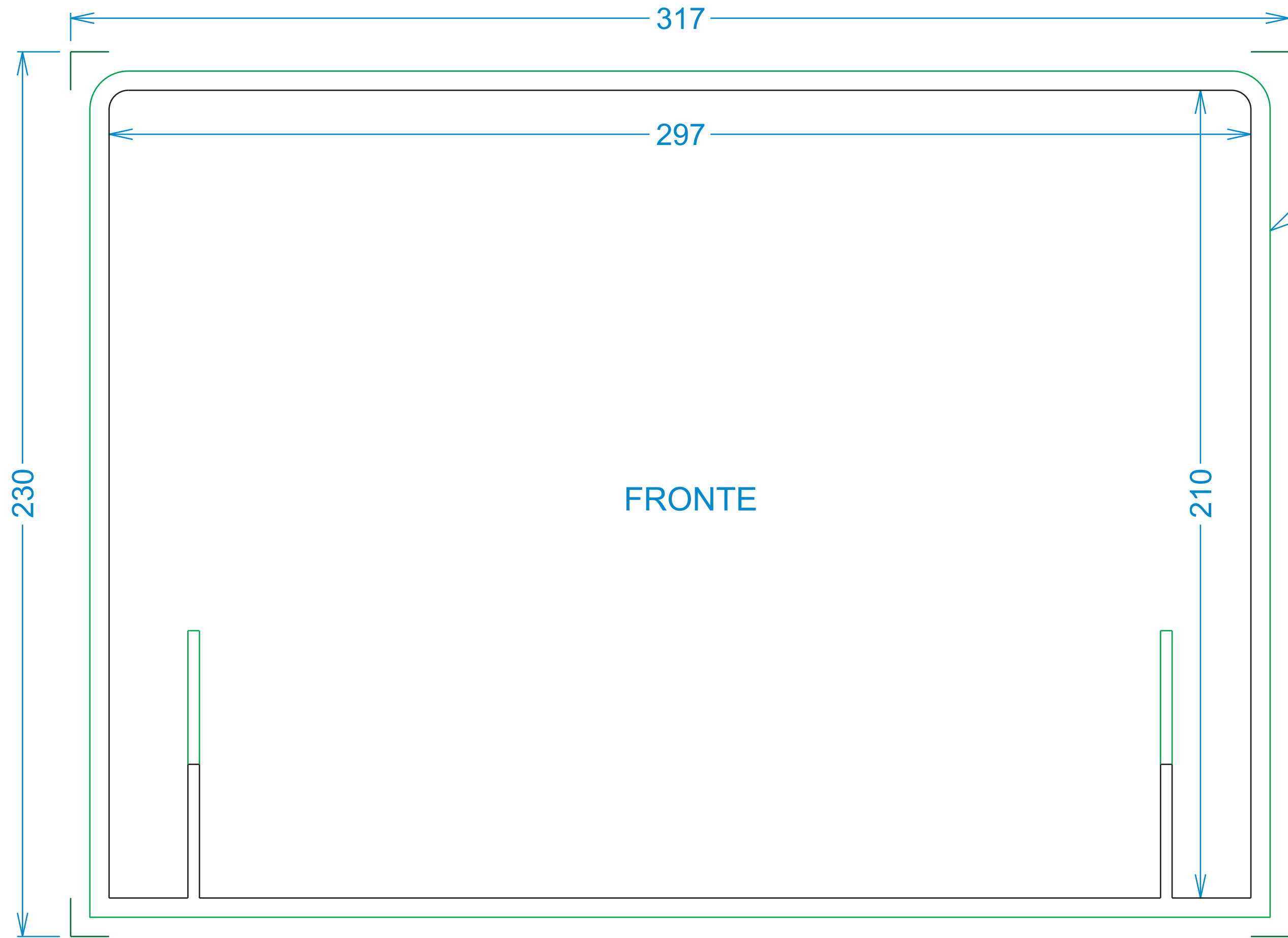
PINZA LATO STAMPA COD. 300_302_3044-01_DIS1
